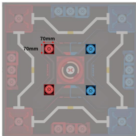
图 4.2-2 中央集散区示意图
