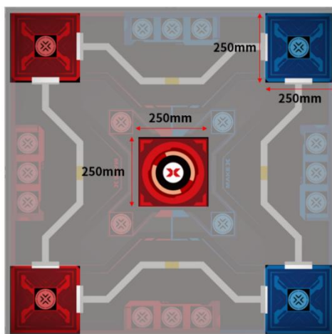
图 4.2-1 基地区/投递区示意图
