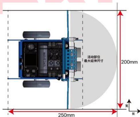
图 5.1-1 最大延伸尺寸俯视图
