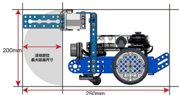
图 5.1-2 最大延伸尺寸侧视图
