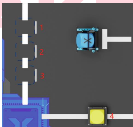
图 4.4-2 M01 任务初始位置示意图
