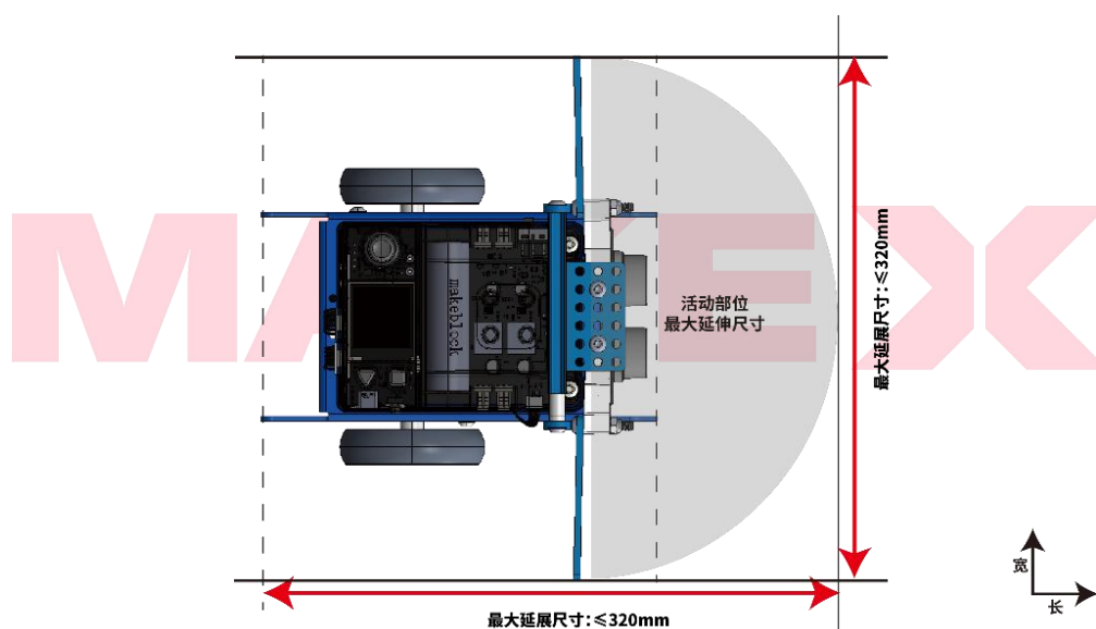
图 5.1-2 最大延伸尺寸-俯视图
