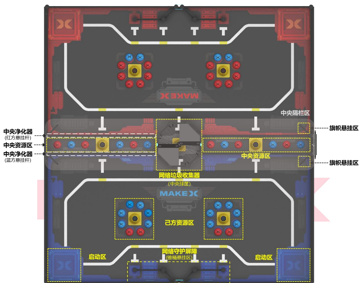
图 4.2-1 场地区域说明图
