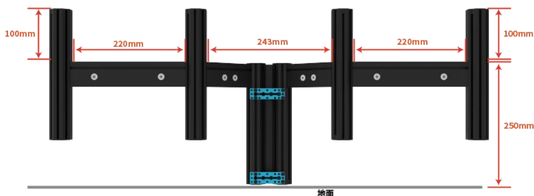
图 4.2-5 锥桶悬挂区示意图
