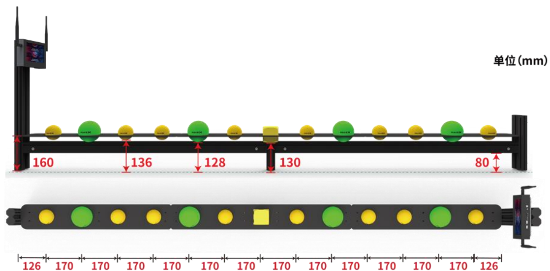
图 4.2-3 CO 2 排放区（中央区）示意图
