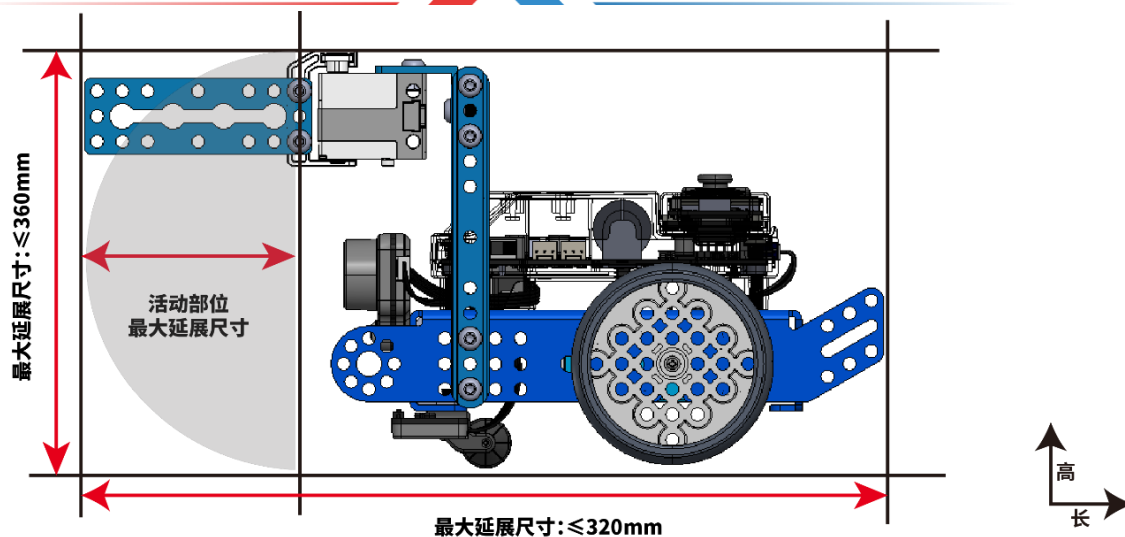
图 5.1-1 最大延伸尺寸-侧视图
