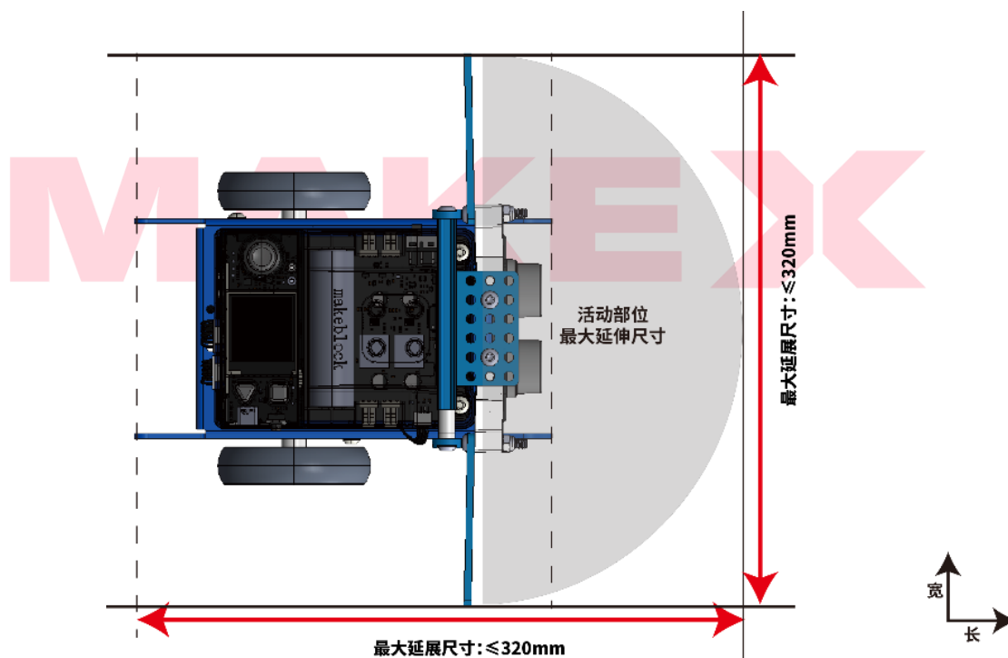
图 5.1-2 最大延伸尺寸-俯视图
